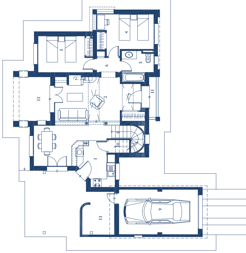
PLANTA BAJA/GROUND FLOOR
